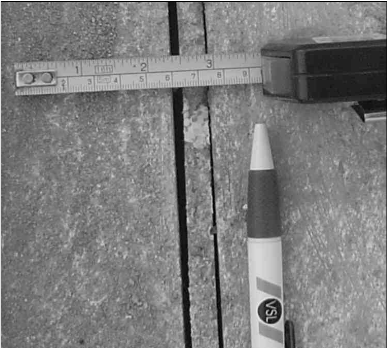
Figura 5: Apertura de una junta observada una semana después del tesado de uno de los paneles.
