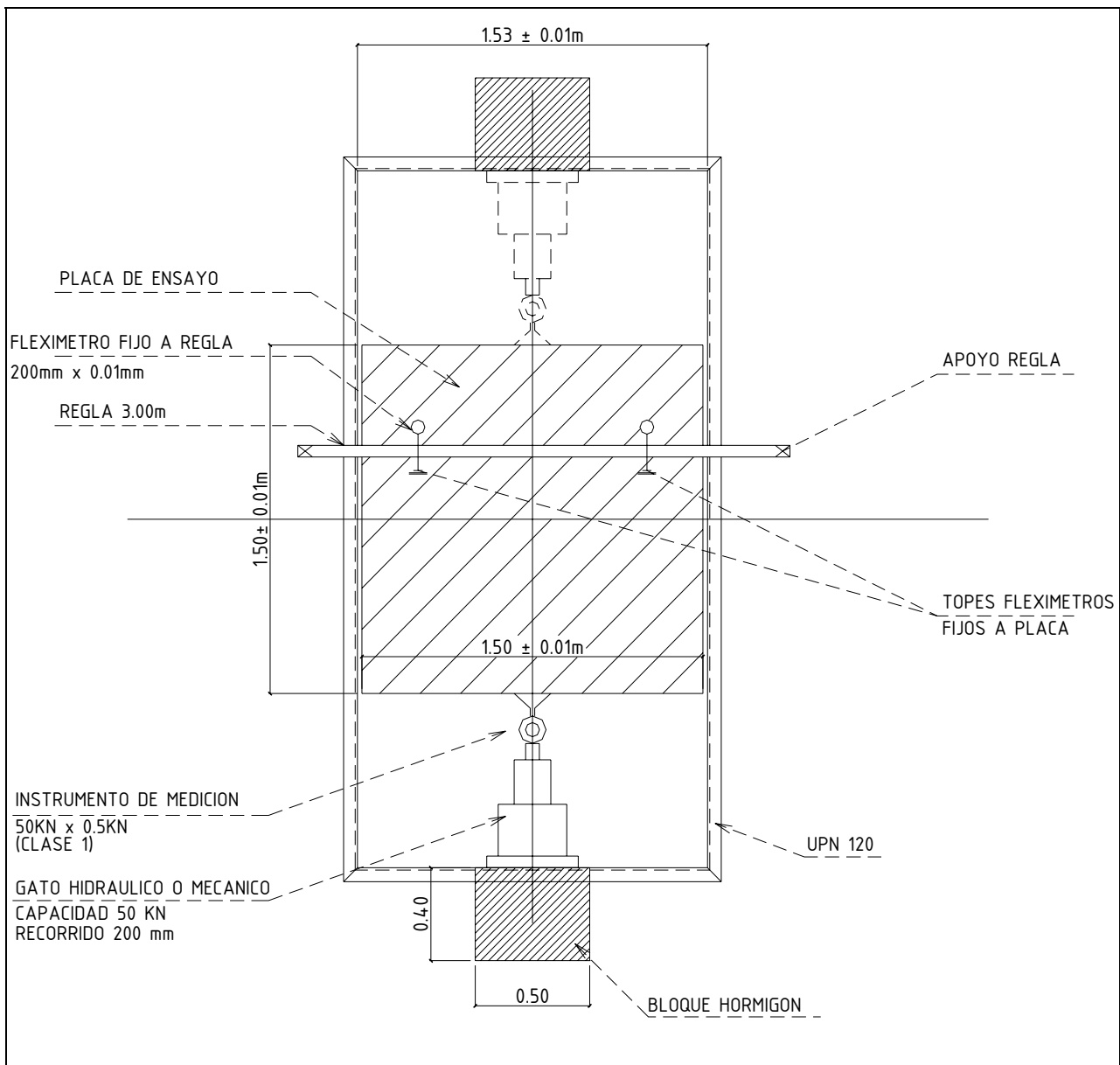
Figura 2: Dispositivo para el ensayo de fricción.
