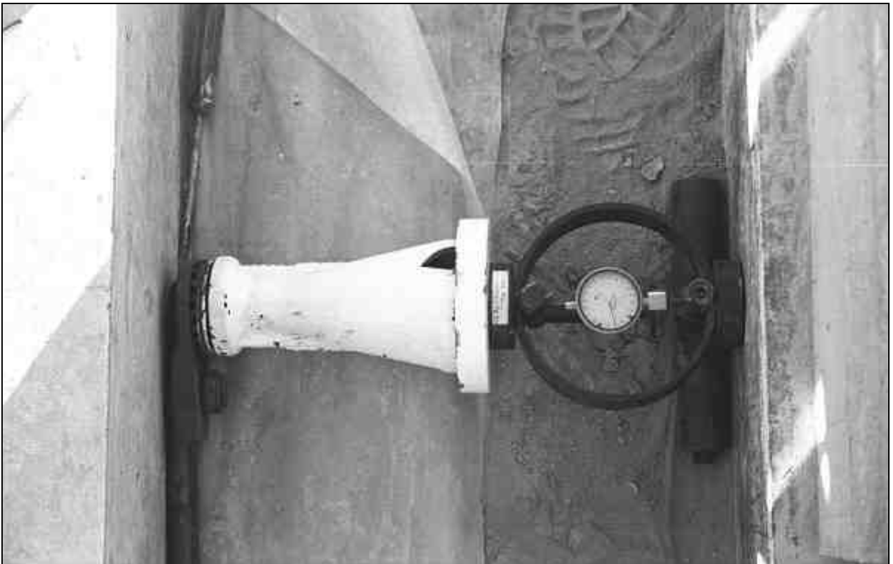
Figura 4: Detalle del gato mecánico que empuja el panel.
